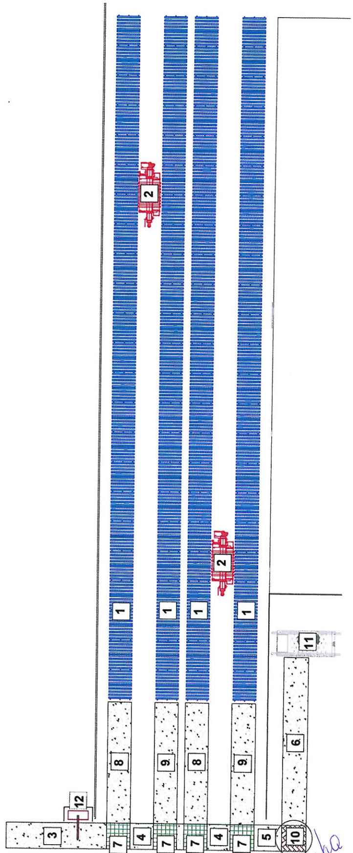
Rys. 1. Rozmieszczenie elementów magazynu automatycznego.
